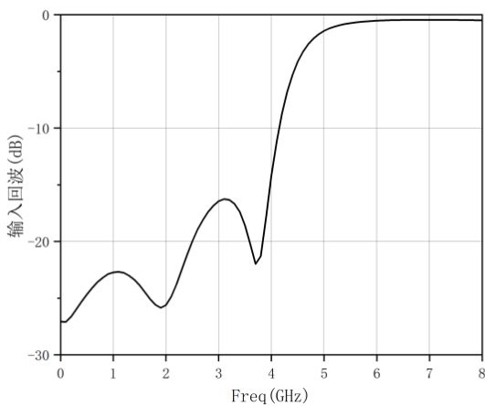
输入回波
